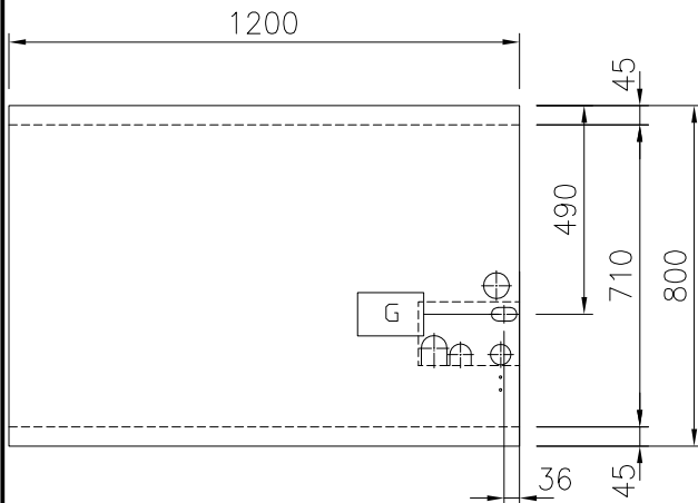
Boven aanzicht
